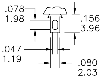
SOLDER LUG
